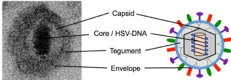
H-particle
